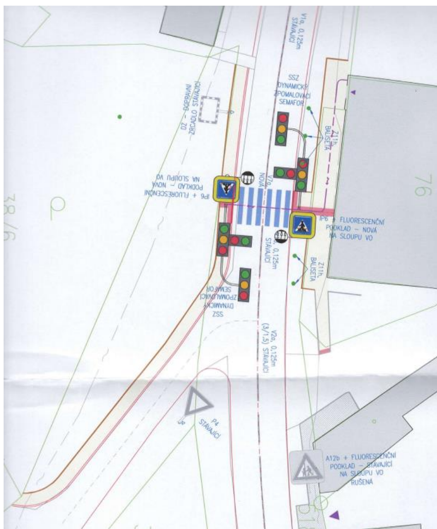
Obrázek 1 – Situační výkres
